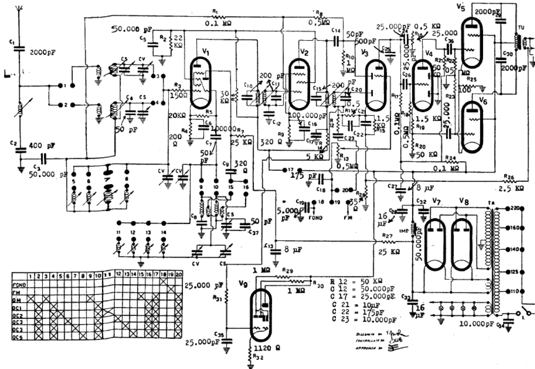
INGAR - Mod. VZ 801 - Onde medie e cinque gamme onde corte. Lo stadio finale è preceduto da un triodo invertitore di fase in circuito catodina. Potenza d'uscita 10 watt.
